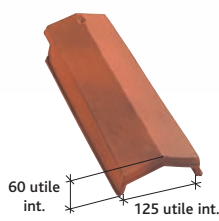
Arêtier Valoise à emboîtement (2,7 au ml) Réf. 310.152
