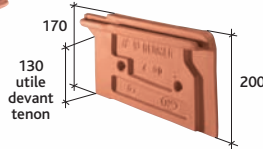
Rive individuelle droite à emboîtement Valoise (3,8 au ml) Réf. 310.41
