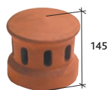
Lanterne petit modèle Ø 100 utile (section d'aération 30 cm²) Réf. 1004
