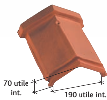
Faîtière Valoise à emboîtement (3,3 au ml) Réf. 310.150
