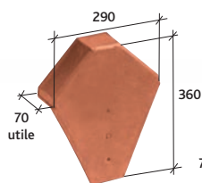
Fronton pour faîtière angulaire à emboîtement (1) Réf. 801
